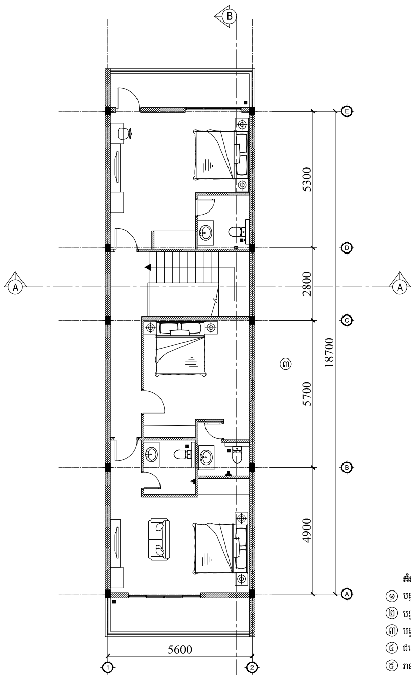
ប្លង់ជាន់ទី១ មាត្រដ្ឋាន១:១៥០
